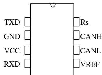
图 1 LM82C251 引脚分布图
