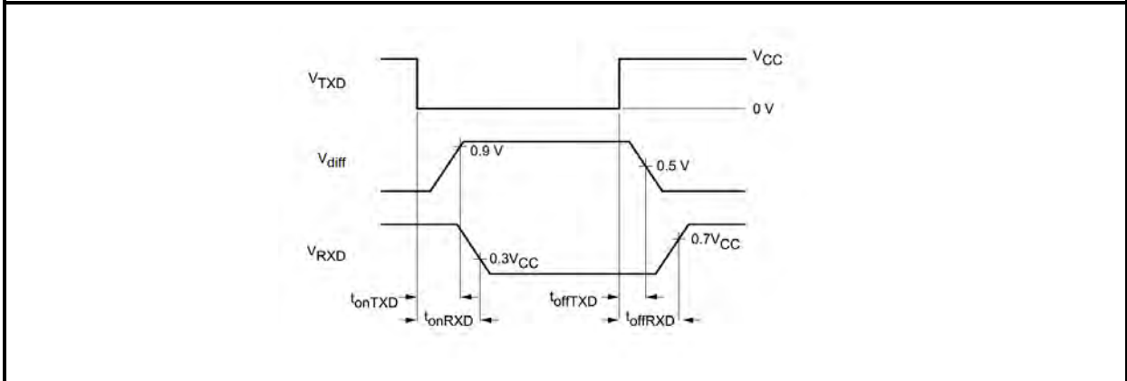
图 3 动态特性时序图
