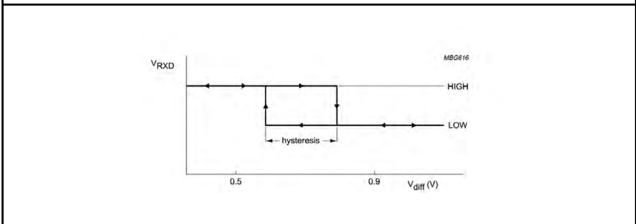
图 4 迟滞
