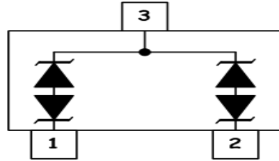
SOT-23
